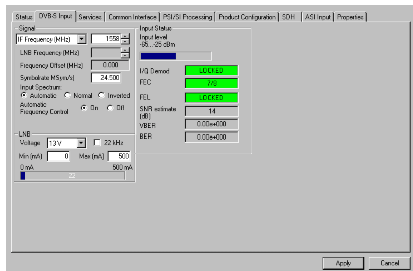
Дисплей Конфигурирования.
