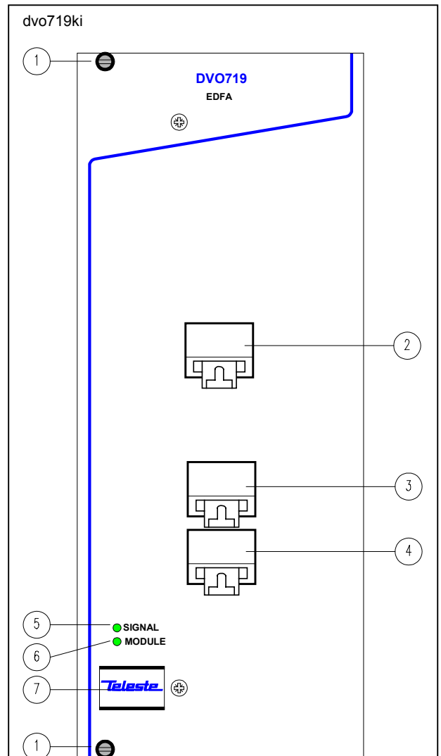
Рис.1. Передняя панель DVO719,
