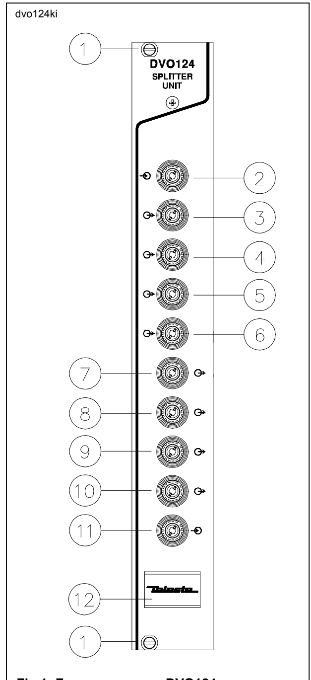
Fig.1. Лицевая панель DVO124,
