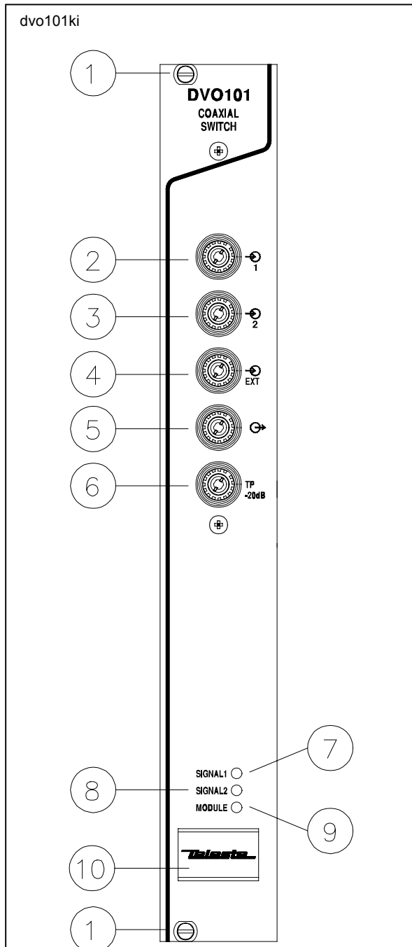
Рис.1.Лицевая панель DVO101,
