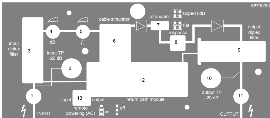
Рис. 4. Места вставок, разъемы и перемычки
