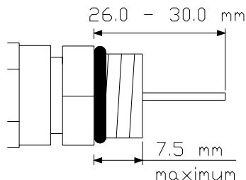
Рис. 2. Длина центрального пина разъема PG11
