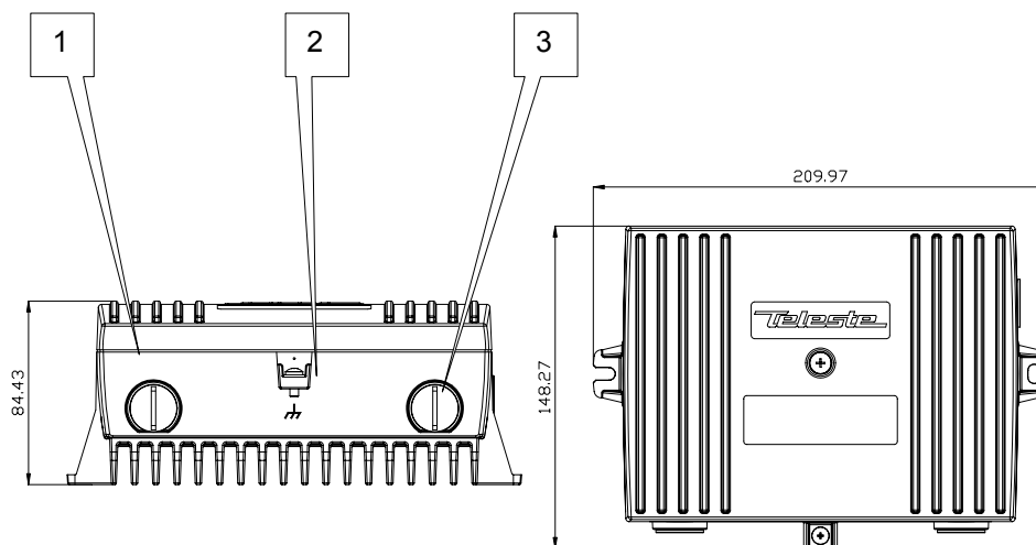
Рис. 1. Усилитель CXE101, 1) вход, 2) заземление, 3) выход
