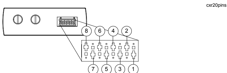
Рис. 5. Разъем транспондера CXR020, 1) земля, 2) земля, 3) земля, 4) аттенюатор обратного канала (-10 дБ), 5) отключение обратного канала (-10 дБ), 6) напряжение дистанционного питания, 7) не используется, 8) +12 В
