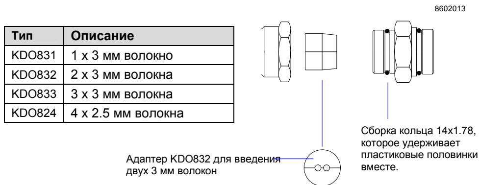
Рис. 4. Адаптеры KDO
